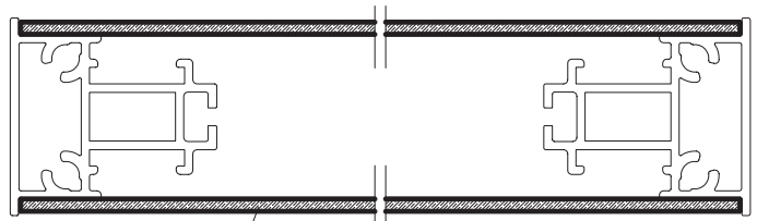
graphic panel max. 3 mm thick - mounted on both sides with glue Grafikpanel max. 3 mm stark - beidseitig aufgeklebt
